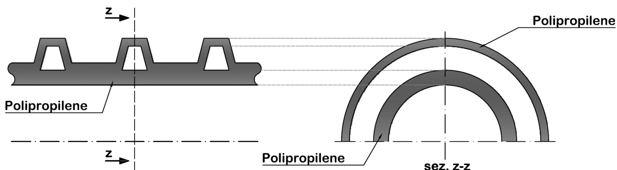
Figura 2. Sezione di una tubazione corrugata a doppia parete (tipo B secondo EN 13476-3:2008).
