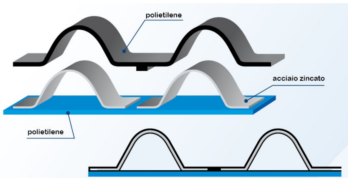
Figura 4. Sezione trasversale del tubo PALADEX.
